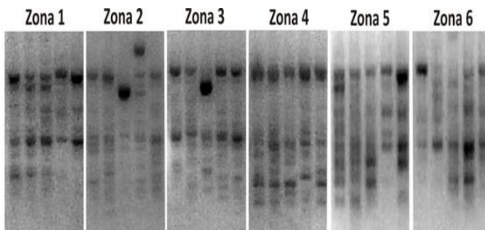
Figura 2. Ampliaciones polimórficas y monomórficas generados mediante el cebador 01 de cinco ejemplares de M. flexuosa procedente de seis zonas de colecta
